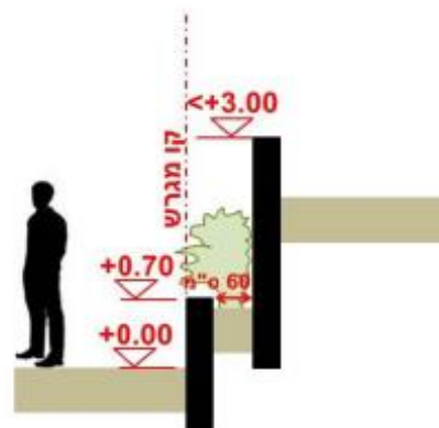
דוגמא לקיר תמך עד גובה 3 מ'
